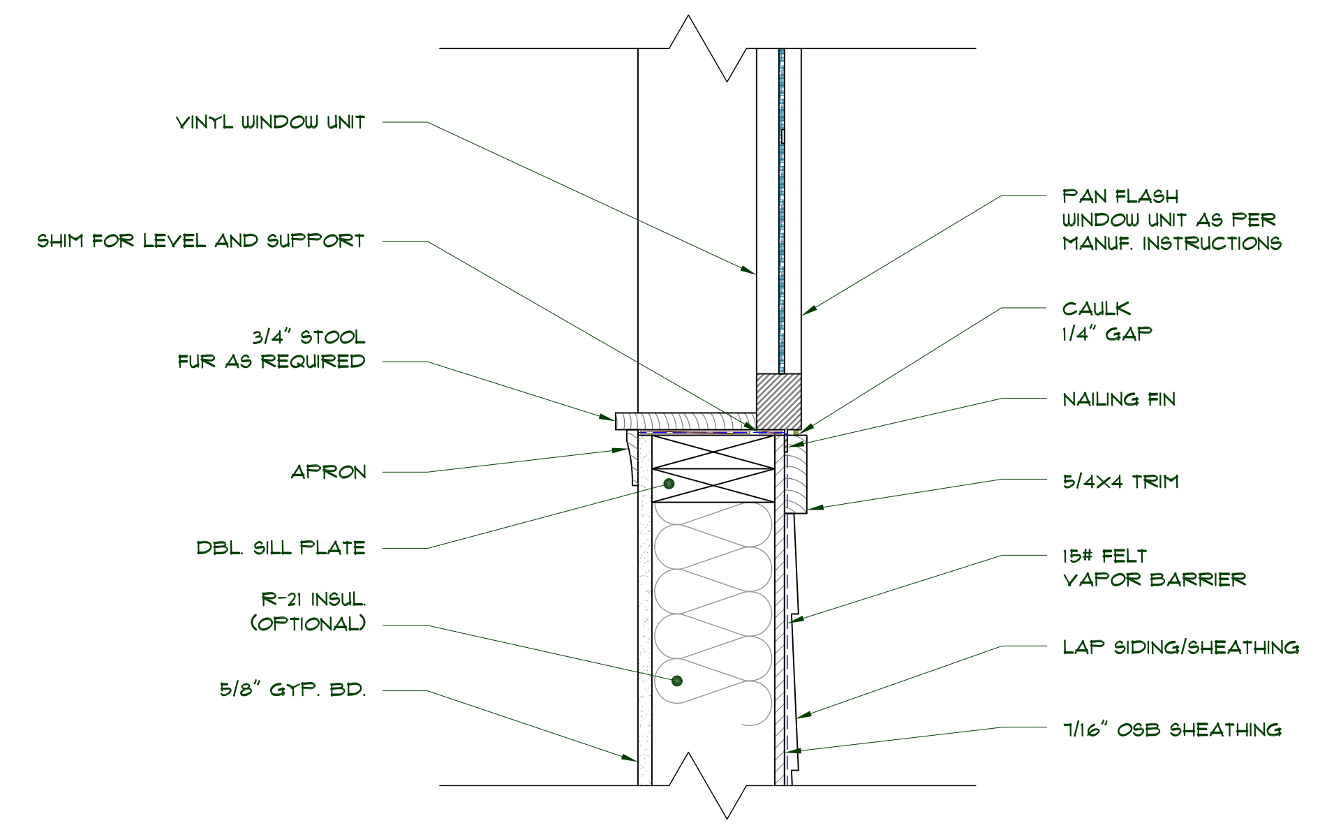
5 WINDOW SILL DETAIL SCALE: 2"=1'-0"
