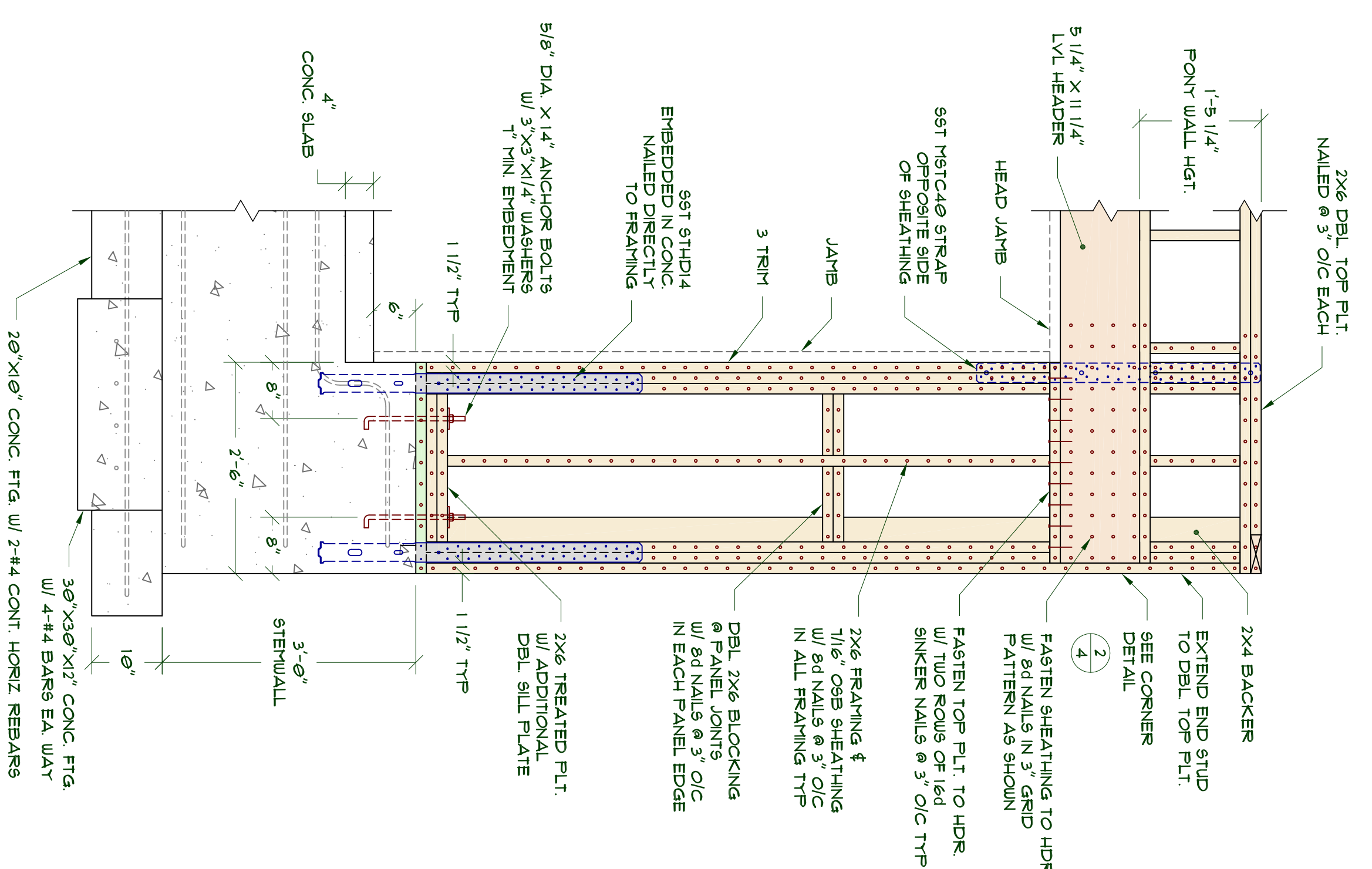
4 GARAGE DOOR END PANEL
